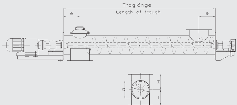
Rohr-schnecken- förderer/ Tubular screw conveyor
