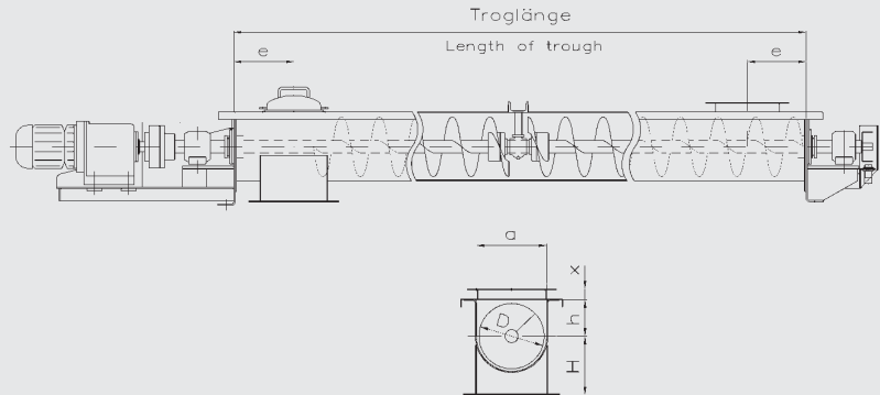
Trog-schnecken- förderer/ Trough-type screw conveyor
